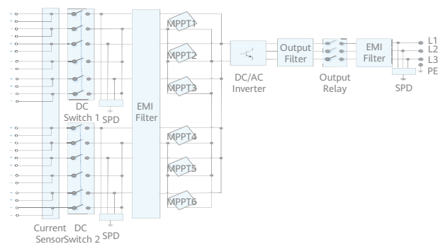
SUN2000-60KTL-M0
